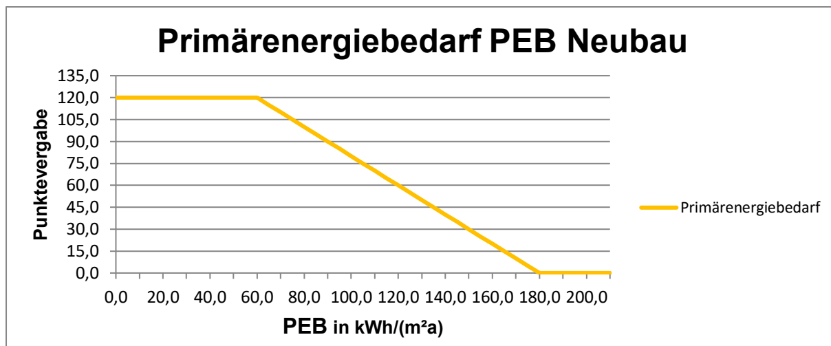
Abb 11: Punktevergabe in Abhängigkeit vom Primärenergiebedarf PHPP beim Neubau
